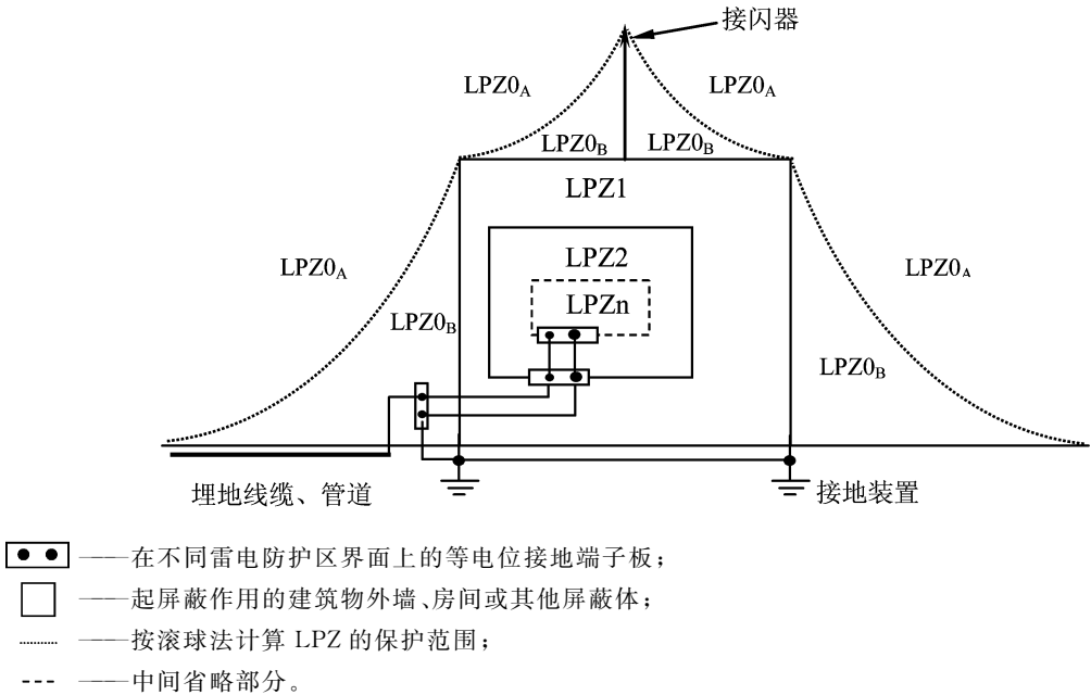
图 B.1 建筑物雷电防护区(LPZ)划分
