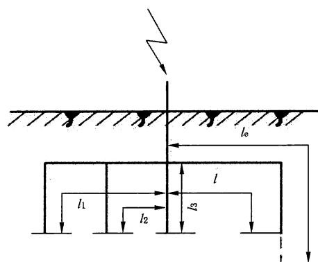
d) 接地根垂直接地体的多根水平接地体, l_1 \leq l, l_2 \leq l, l_3 \leq l
