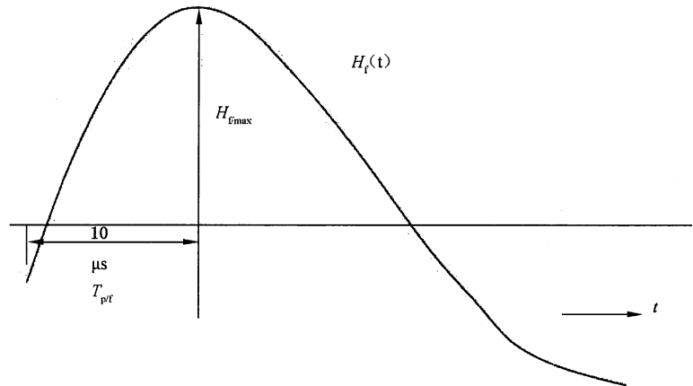
图 F.3 首次雷击磁场强度(10/350 \mu s )上升期的模拟
