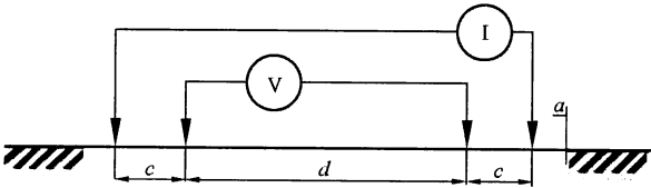
图 B.2 电极非均匀布置
