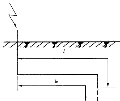
b) 末端接垂直接地体的单根水平接地体
